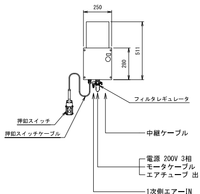
制御ボックス
