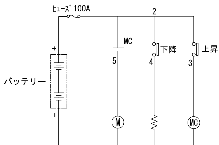
電気回路図
