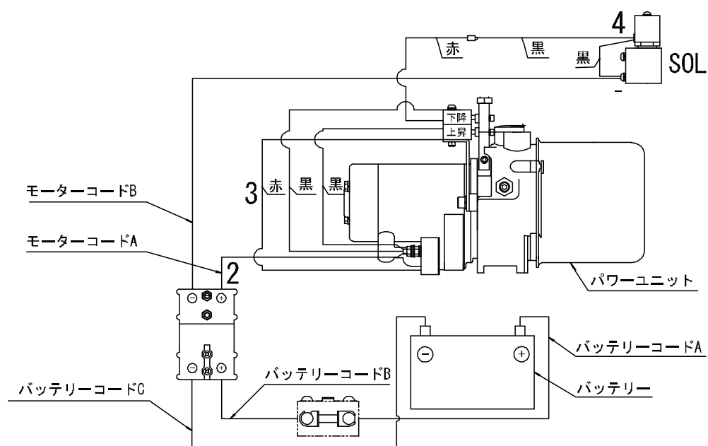
実態配線図
