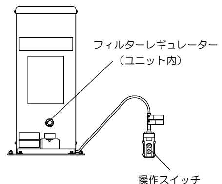
＜別置油圧ユニット（床置き式）＞ ※制御盤一体型
