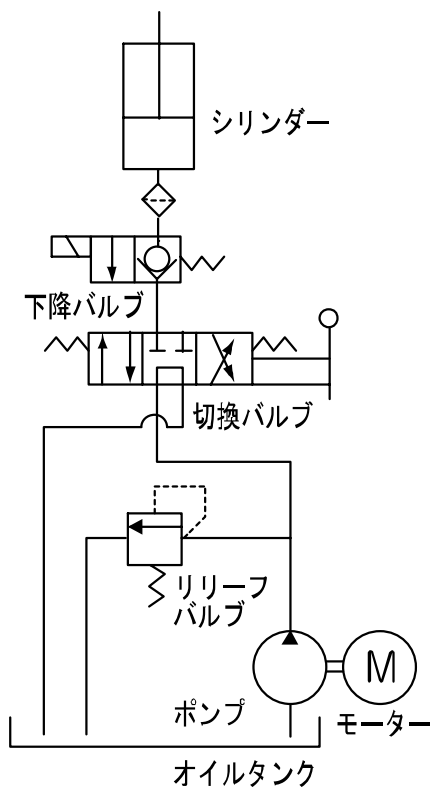
油圧回路図
