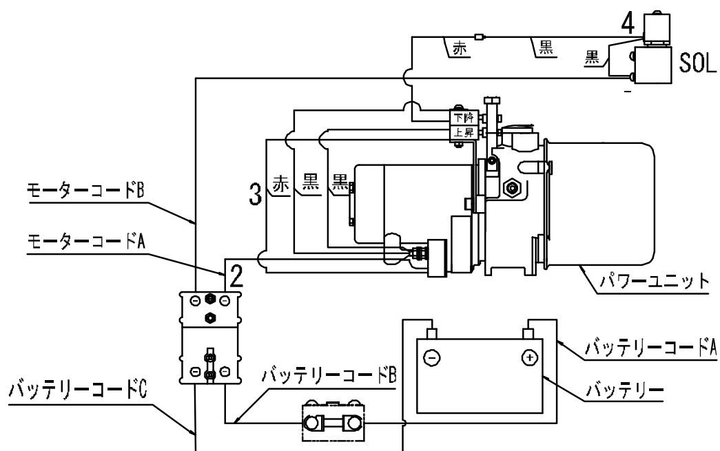
実態配線図
