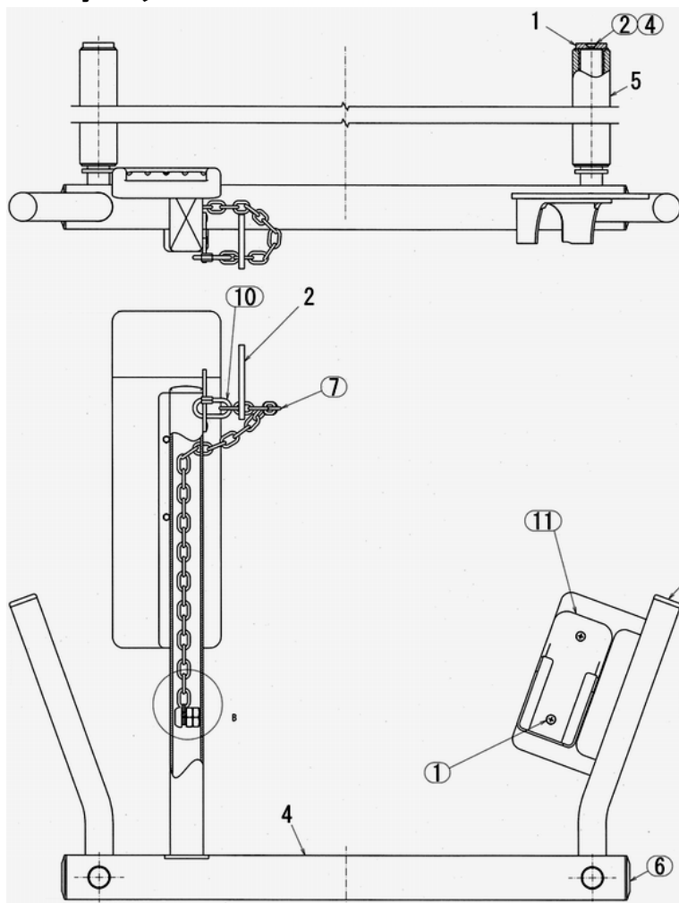
図番7-5 回転フォークAS
