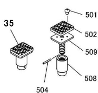
フレームアタッチメントLB AS
