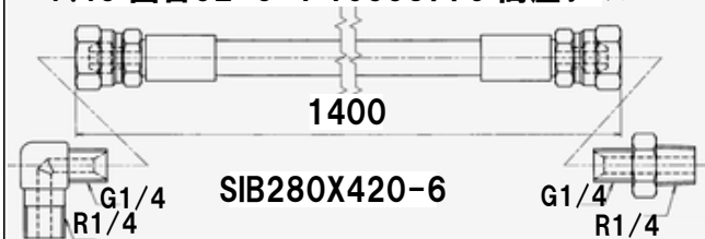
P.43 図番52-6-1 10398770 高圧ホース
