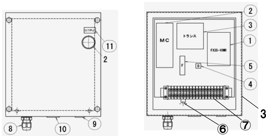
図番25-1-1 制御ボックスAS (ユニット内蔵式)
