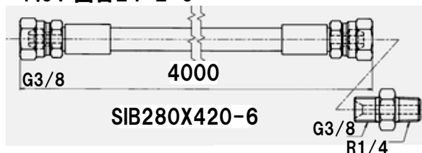
P.43 図番52-6-1 10398770 高圧ホース
