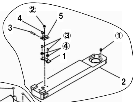
図番13-5-02-2 受台ベースBAS
