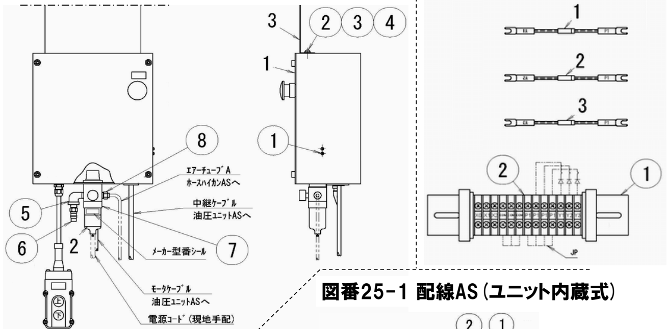
図番25-1-2 端子台AS
