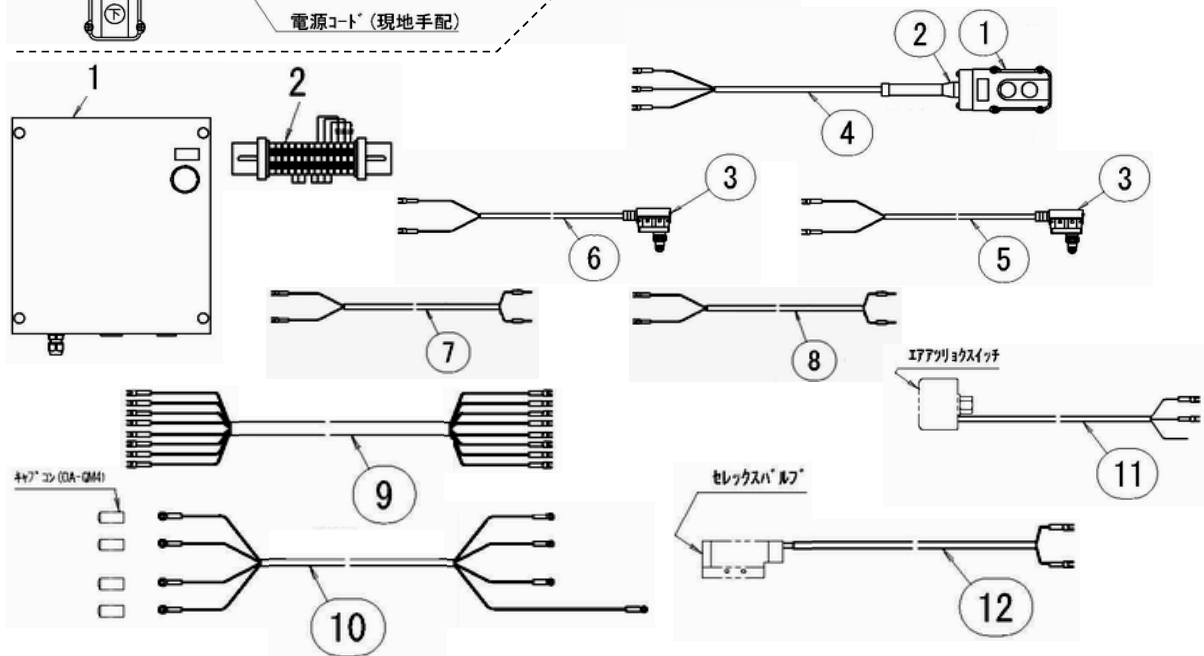
図番25-1-1 制御ボックスAS (ユニット内蔵式)
