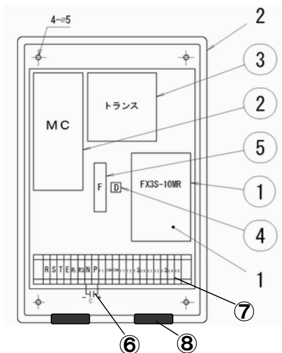
図番52-9-2 別置式制御ボックスAS
