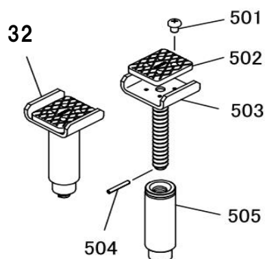
旧型フレームアタッチメントHAAS
