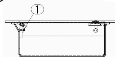
図番19・20 A方向詳細図
