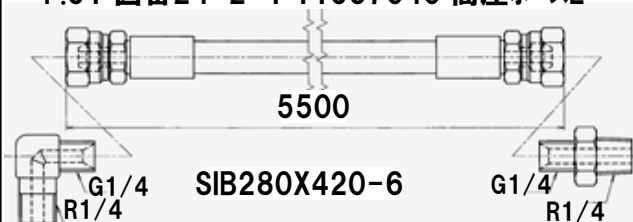
P.51 図番24-2-1 11537040 高圧ホースL
