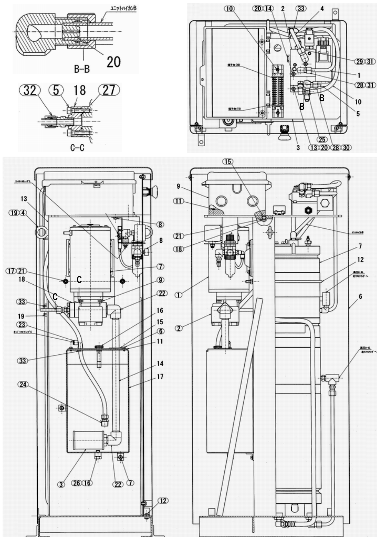
図番52 別置式油圧ユニットAS
