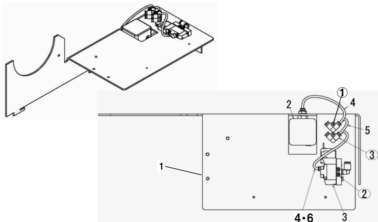
図番17-9-2 エア圧力スイッチAS
