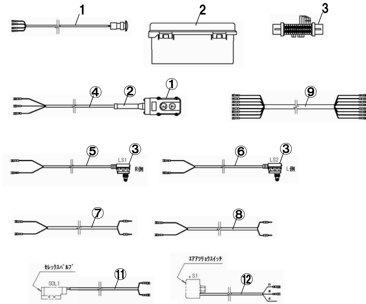
図番52-9 別置式配線AS
