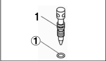
図番52-8-9 ロワーリングAS
