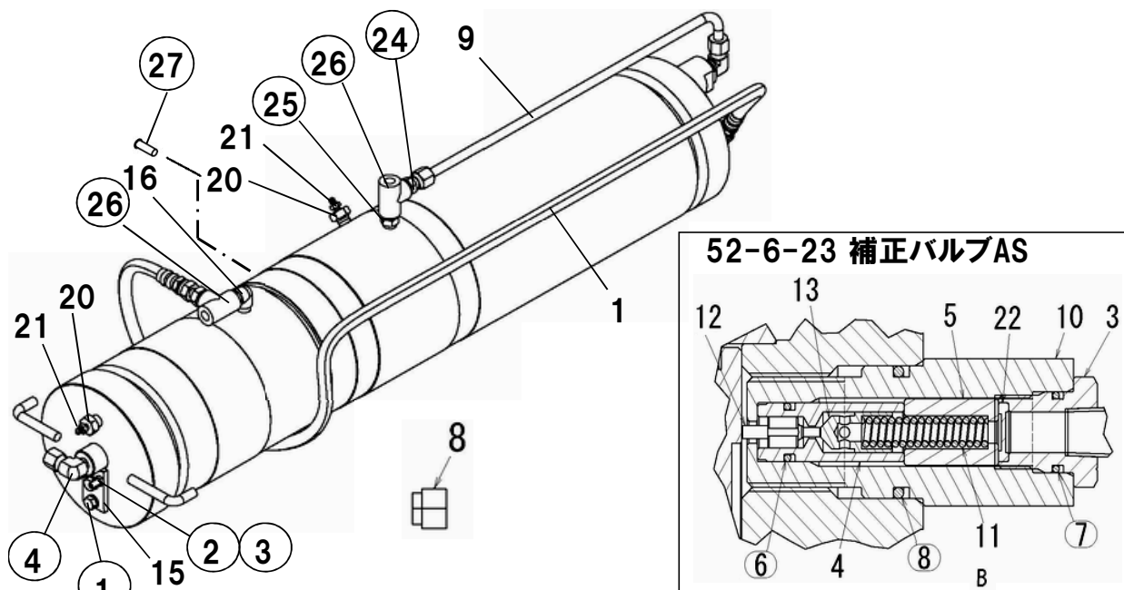
図番52-6 別置式シンクロシリンダAS
