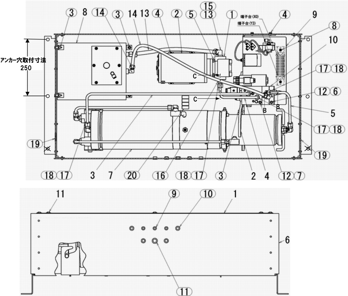
図番17 内蔵式油圧ユニットAS
