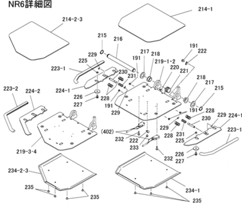
NR6詳細図
