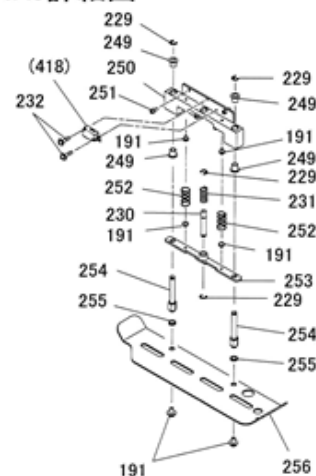
NR5詳細図
