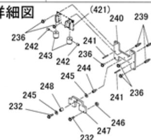
NR5詳細図
