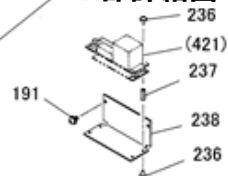
A部詳細図
