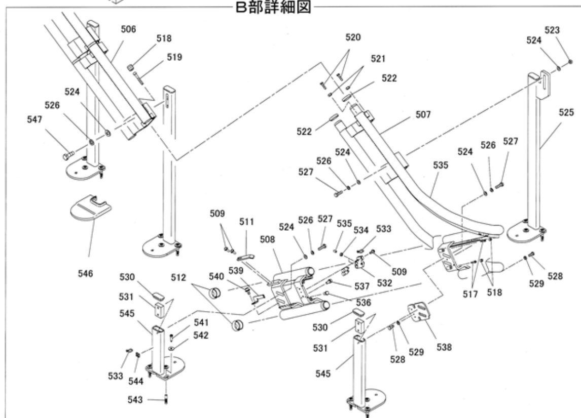
B部詳細図
