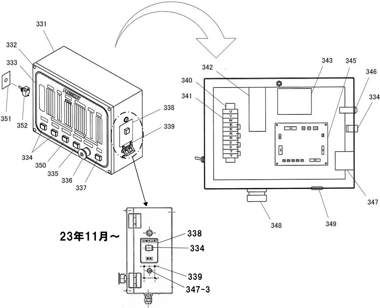
制御ボックス内部
