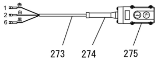
272 (押釦スイッチAS) 詳細図
