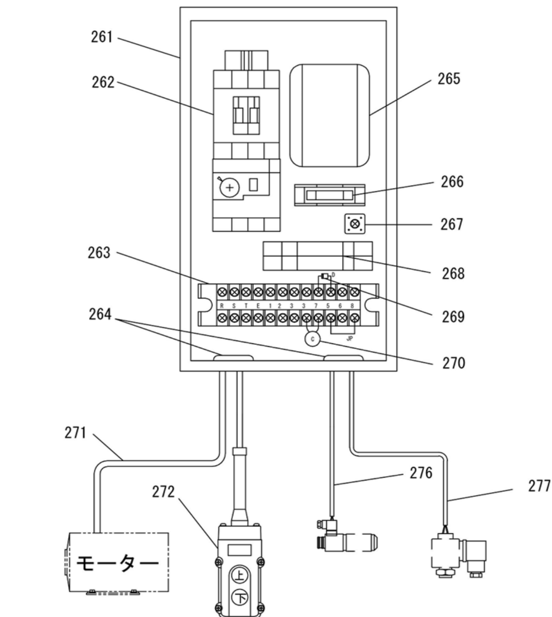
271 (モーターケーブルセット) 詳細図
