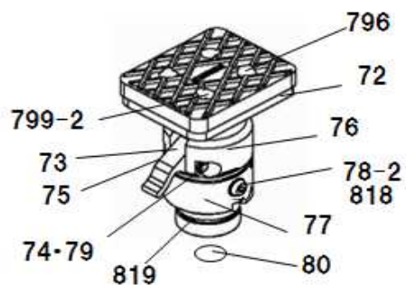
図番U-04 イーザーアタッチメントLB AS (オプション)
