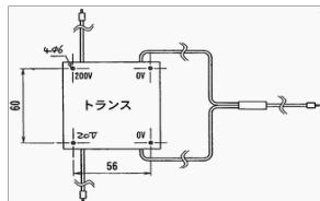
図番585 トランス接続方法
