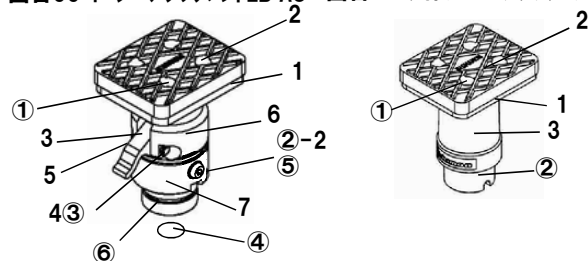
図番39 イーザーアタッチメントLB AS 図番41 ライトフレームアタッチメントLB AS
