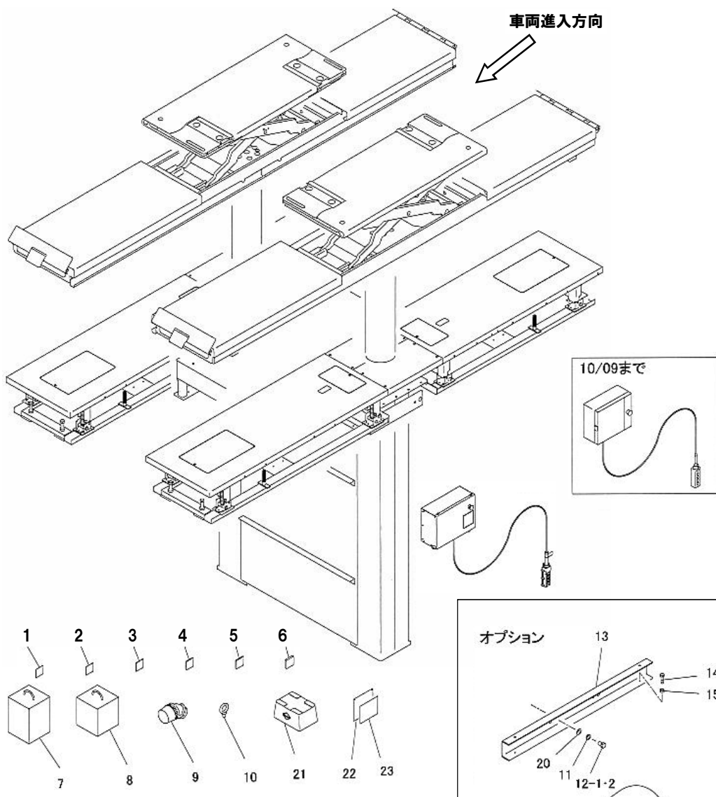
図番39 イーザーアタッチメントLB AS 図番41 ライトフレームアタッチメントLB AS
