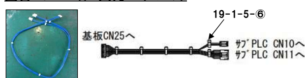
図番19-2-⑨ ツイストペアケーブルセット
