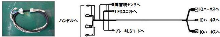
図番19-1-2 ハンドルハーネスセット
