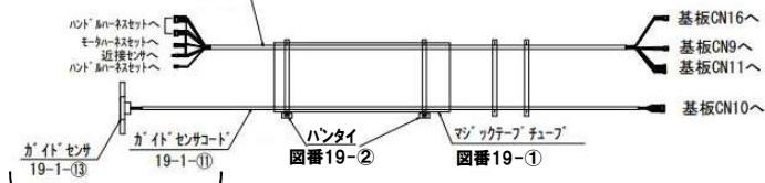
図番ABM10 ガイトセンサAS
