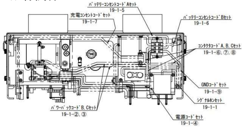
ヒューズ' 端子台 コンタクタ間 配線詳細図
