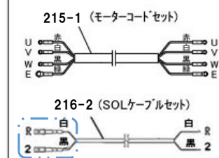
配線詳細図
