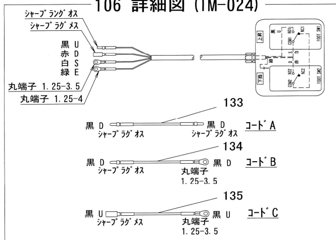
106 詳細図 (TM-024)
