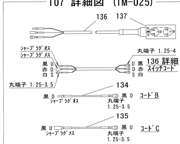
107 詳細図 (TM-025)
