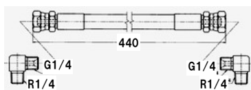
図番28-3-1 11221820 高圧ホースA SIB210-6
