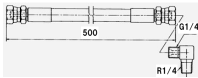
図番28-3-2 11222340 高圧ホースB SIB210-6
