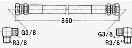
図番28-5 11225520 高圧ホースA SIB210-6
