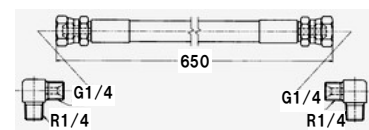
図番28-2-2 12892000 高圧ホース SIB210-6
