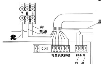
ハンドル'ループ'AS配線詳細図
