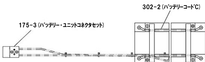
バッテリー結線説明図
