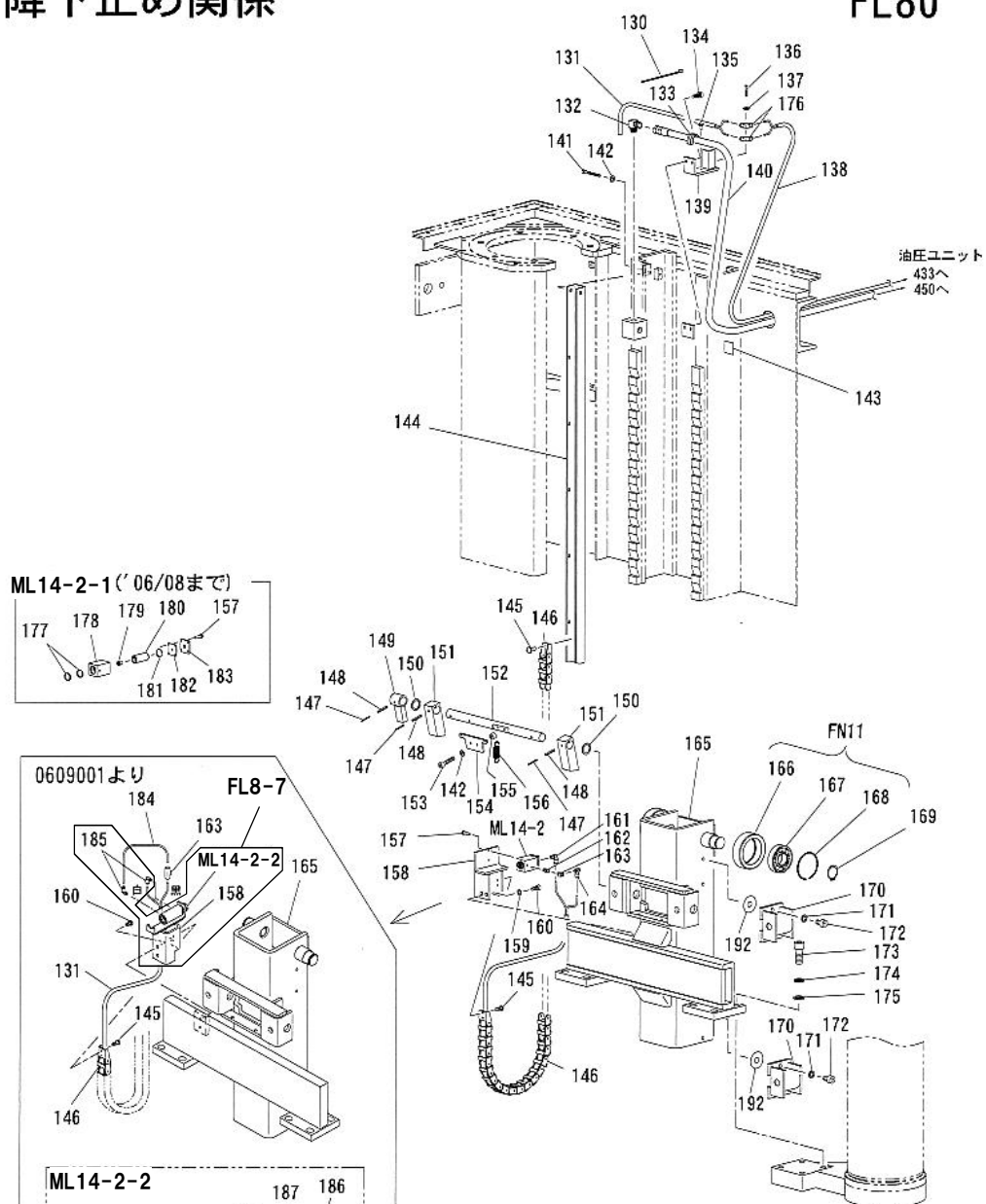
図番140-1・243 (P15) (11019180) 高圧ホース
