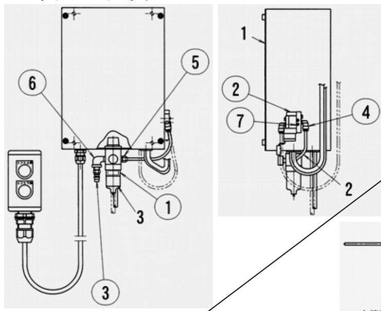
図番18 制御ユニットAS
