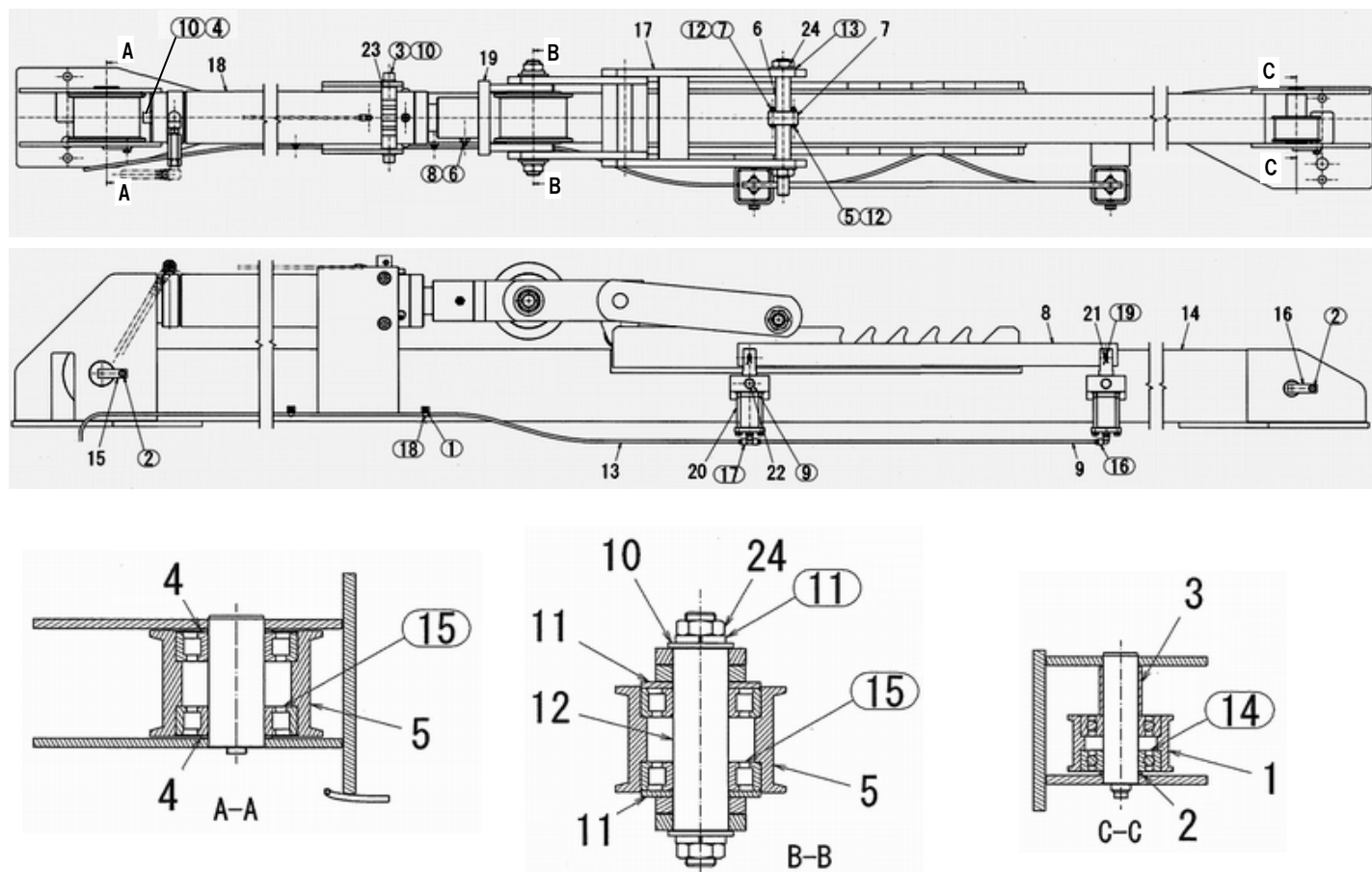
図番13 ポストビームAS
