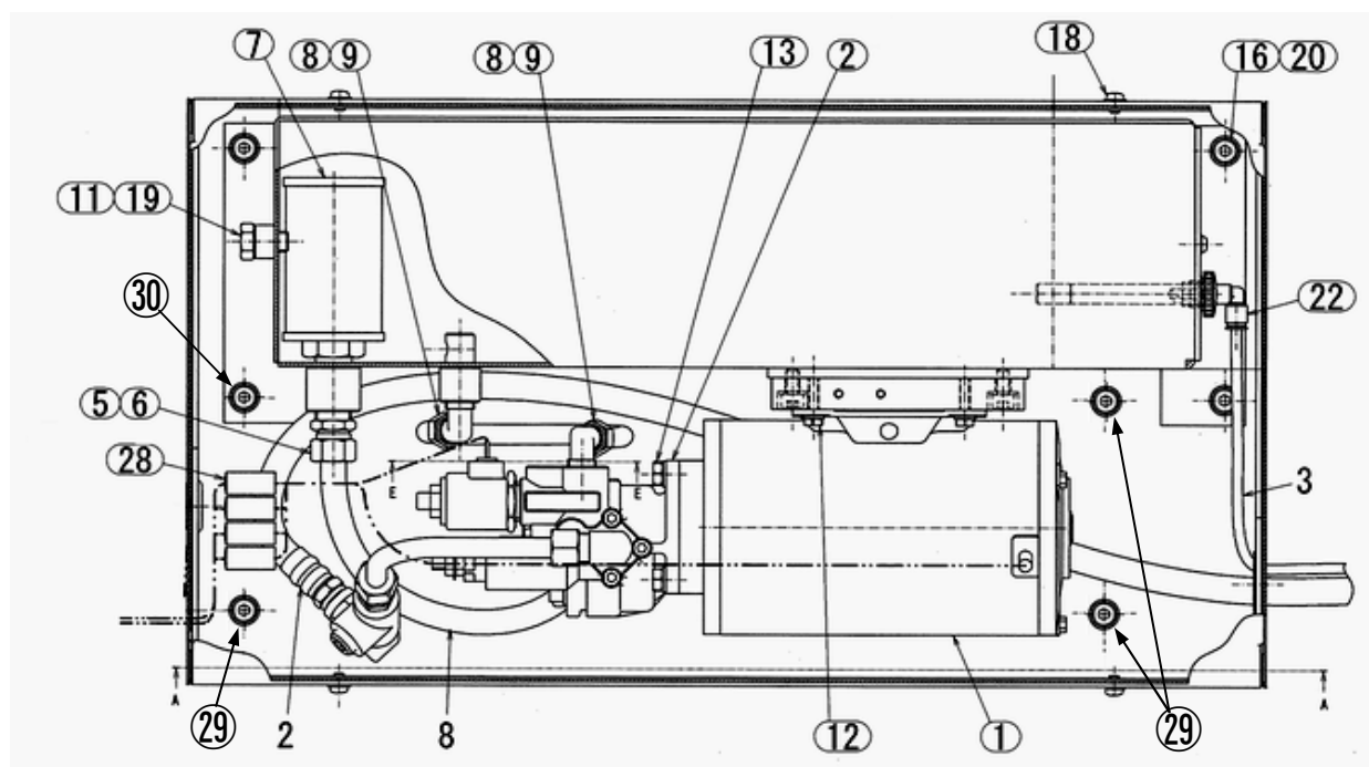
図番17 油圧ユニットAS
