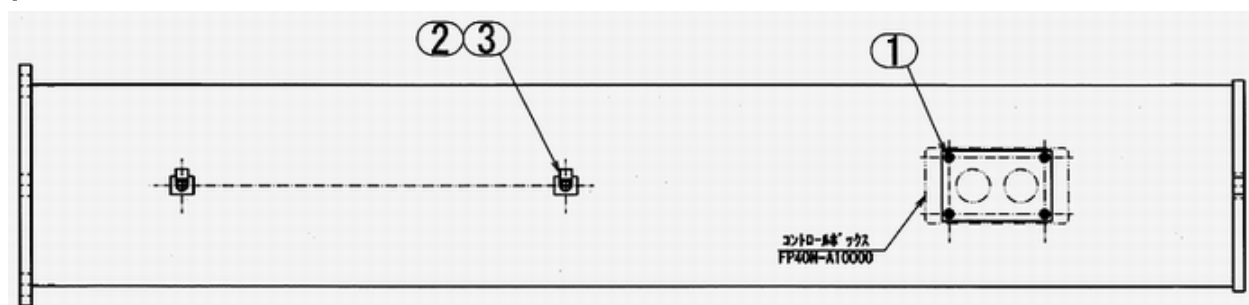
図番12 SポストBAS
