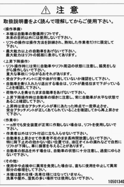
図番7 注意シール
