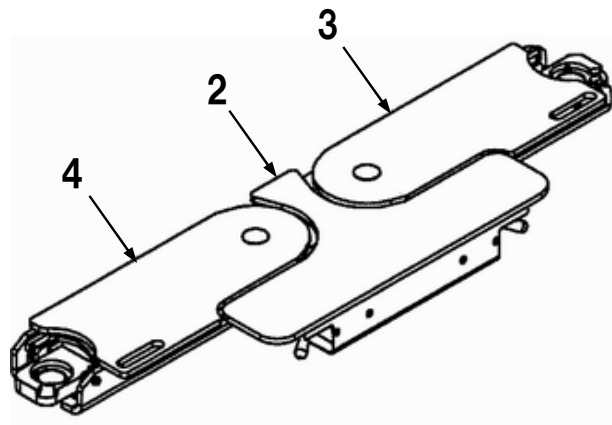
図番4 受台RAS
