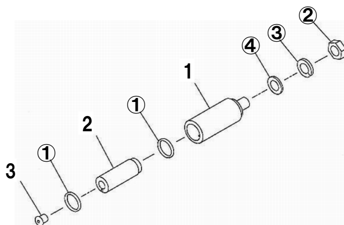
図番3-6-6-2 爪外しシリンダAS
