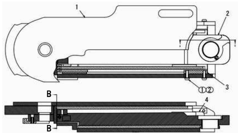
図番4-4 アームLAS
