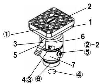
図番24 ライトフレームアタッチメントLB AS
