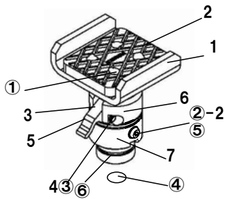
図番21 イージーアタッチメントLA AS
