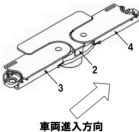
図番5 受台LAS
