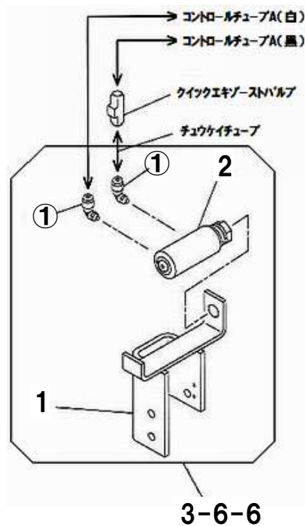
図番3-6-6 爪解除AS
