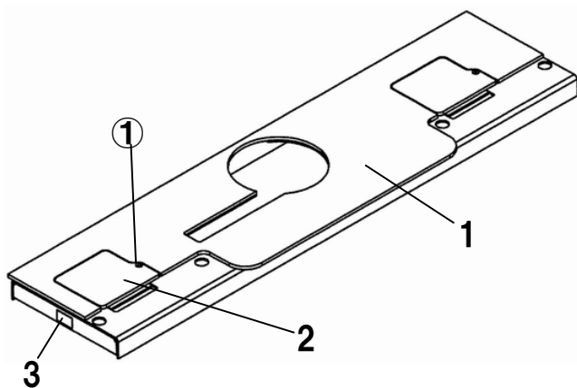
図番10 ボックスカバー-AAS
