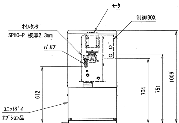
油圧ユニット オプション装着品
