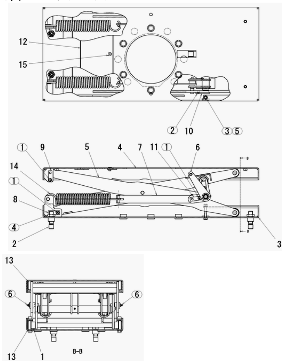
図番4 フラットキットRAS
