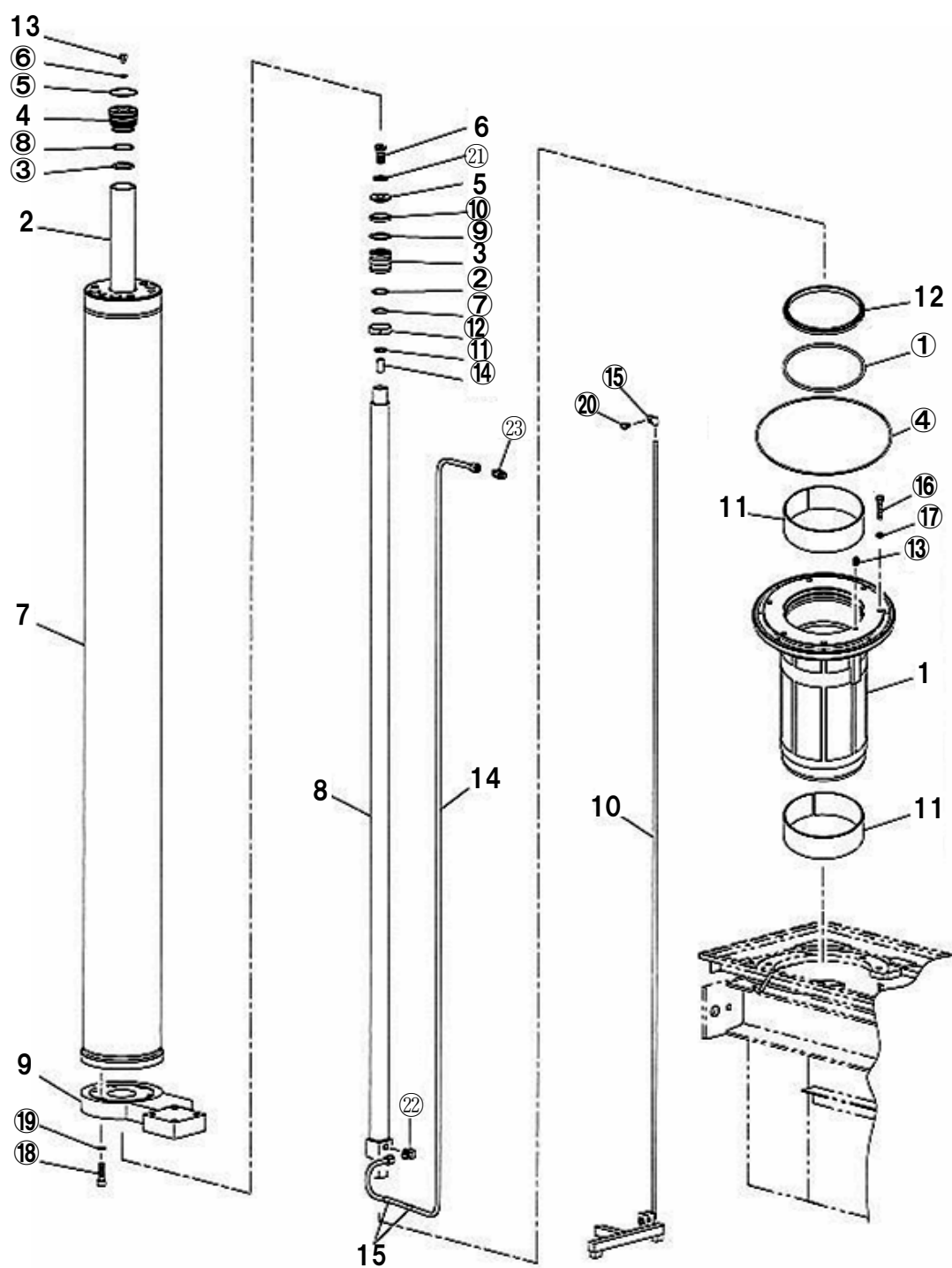
図番8-5 Lラム本体AS
