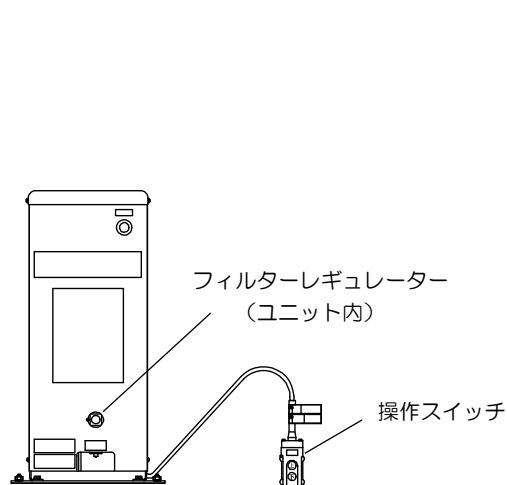
＜別置油圧ユニット（床置式）WAL30WP＞
