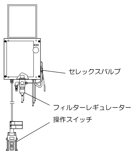
＜制御ボックス（壁掛式）AL30WPU＞
