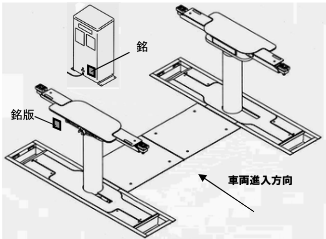
NNZ40WP 進入方向左側受台側面・ユニットケース正面下側
