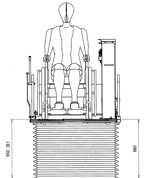
<最大負荷時>
