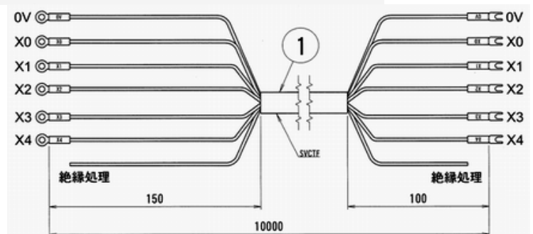
図番9-1-3 中継端子台AS
