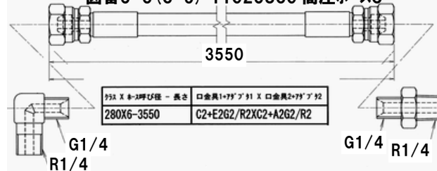
図番5-3 (6-9) 11025860 高圧ホースC
