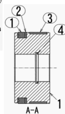
図番6-3-3-6 MSピストンAS
