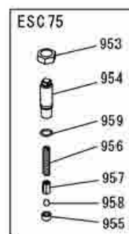
図番5-1 (6-8) 11025840 高圧ホースA
