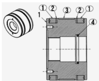
図番5-12-10-6 MMピストンAS
