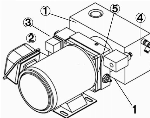
図番10-10 パワーパックAS
