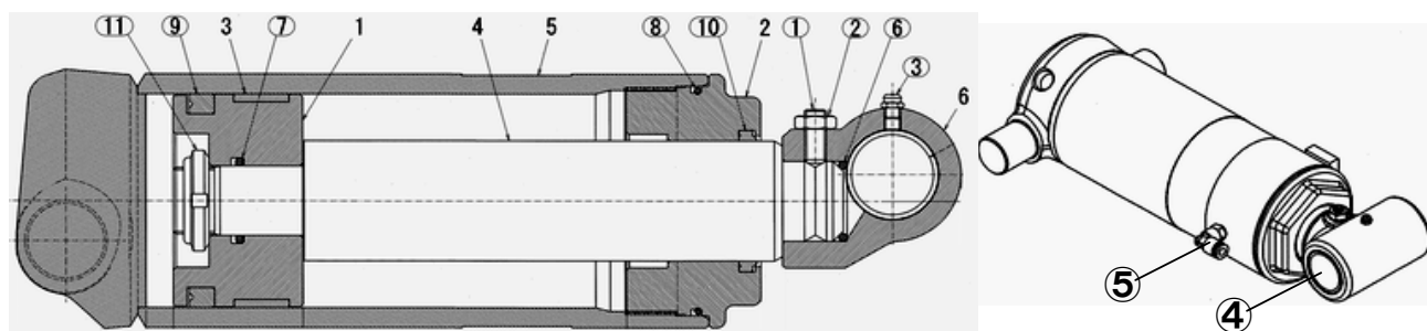
図番10-6 テーブルシリンダAS
