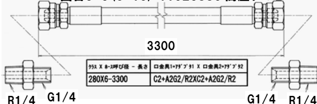
図番5-5 (6-10) 11025880 高圧ホースE
