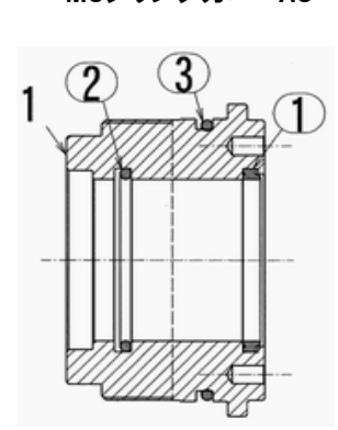
図番6-3-3-7 MSシリンダカバーAS
