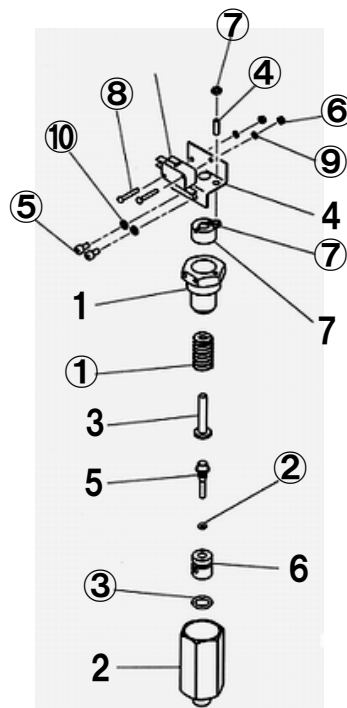
図番8-1-8 圧カスイッチAS
