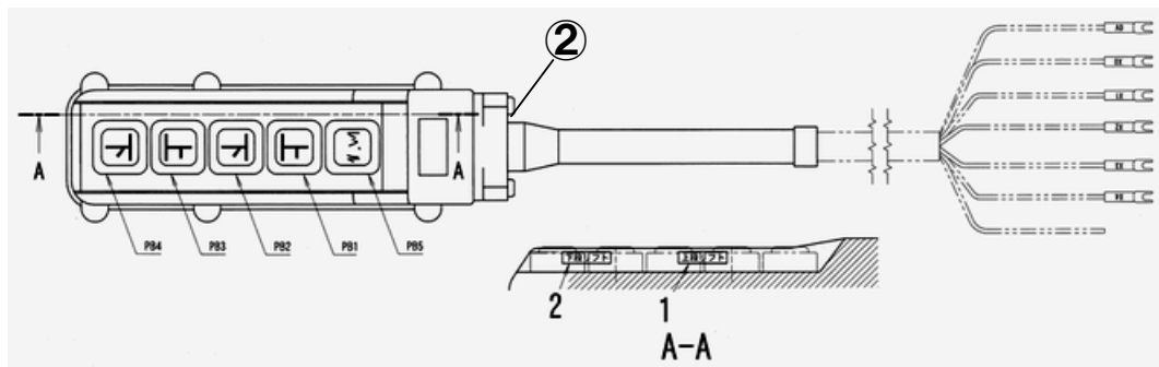
図番9-1-2 押ボタンスイッチAS
