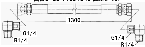
図番5-22 11034040 高圧ホースH
