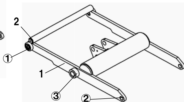
図番10-5 アウターアームAS
