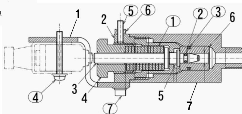
図番8-1-9 下段圧カスイッチAS
