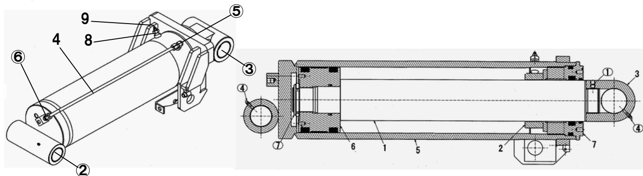
図番5-12-10-6 MMピストンAS
