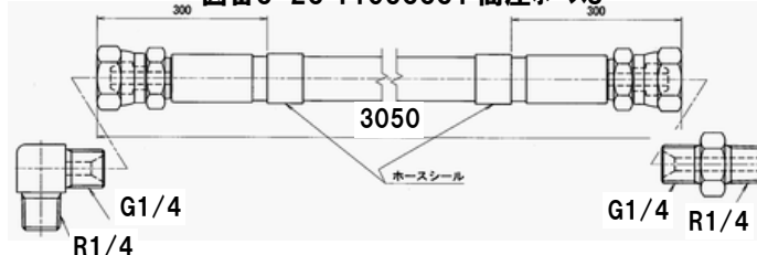
図番6-26 11036661 高圧ホースI
