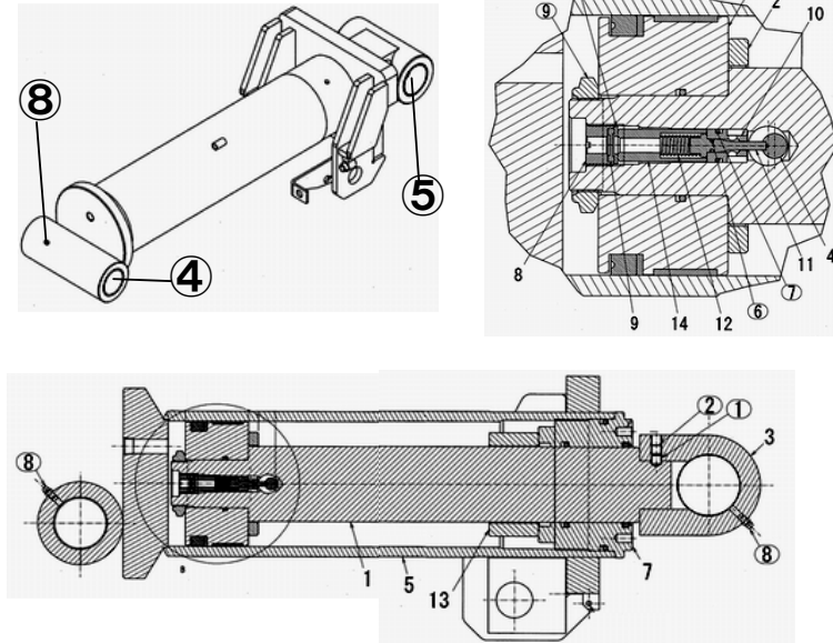
図番6-3-3 MSシリンダAS
