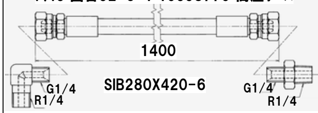
P.43 図番52-6-1 10398770 高圧ホース
