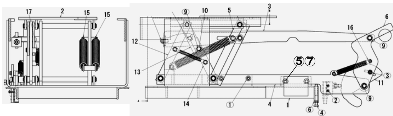
図番8-2-3 連結リンクLAS
