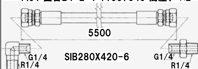
P.51 図番24-2-1 11537040 高圧ホース
