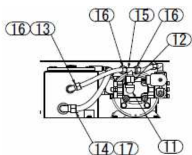
A-A (1 : 5)
