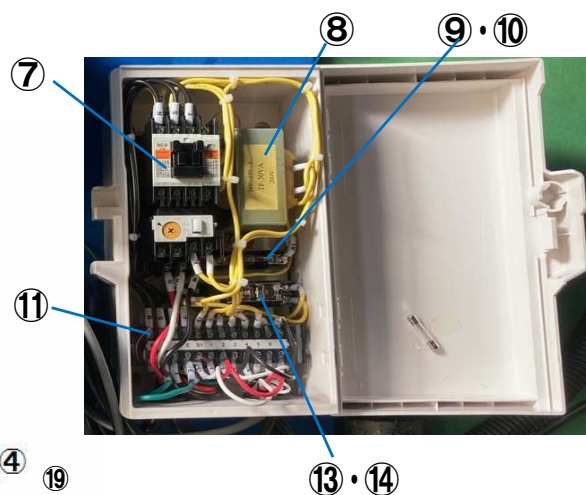
制御ボックス内部詳細図
