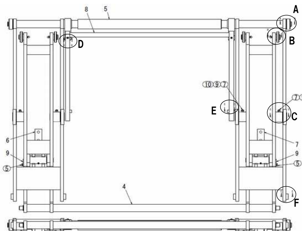
図番17 リンクAS
