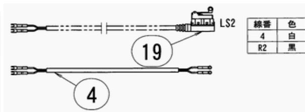
制御ボックス内部詳細図
