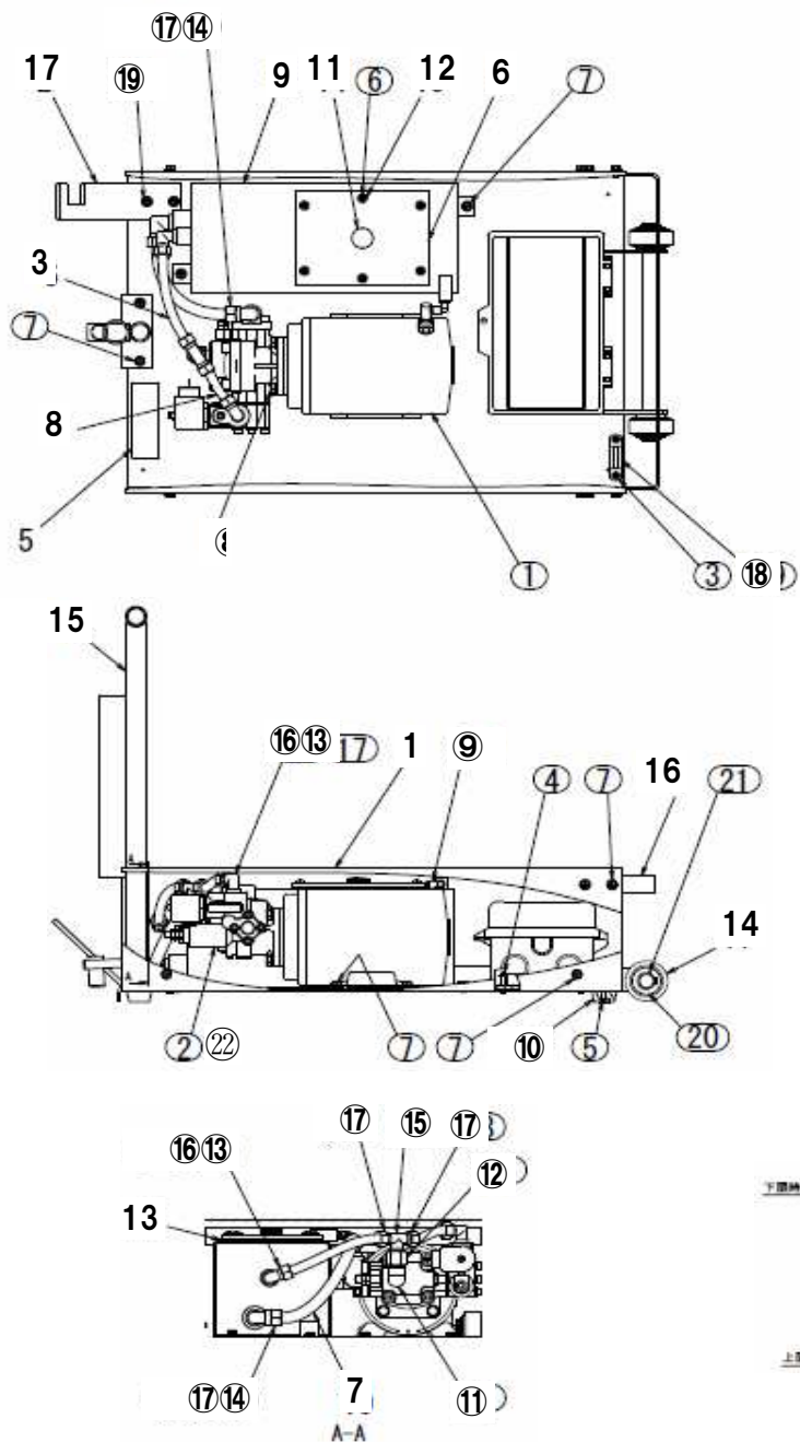
図番36 移動ハンドルAS
