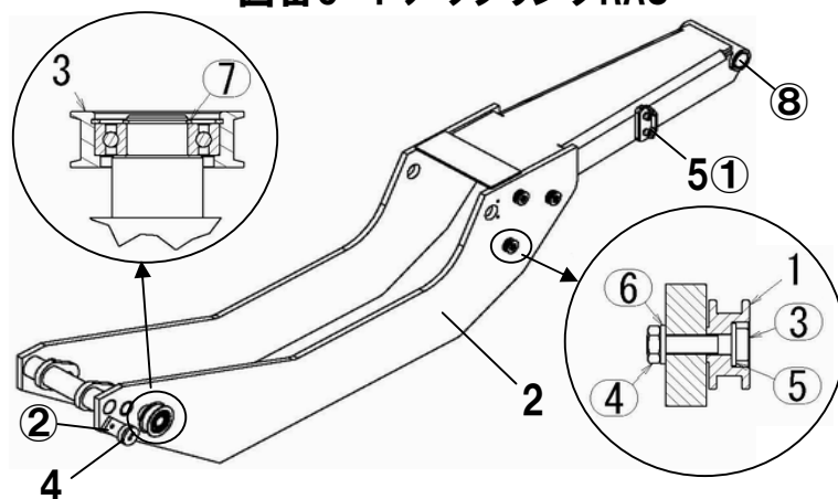
図番9-1 アウタリンクRAS
