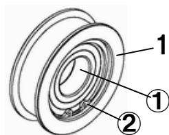
図番9-1-3 ガイドローラAS
