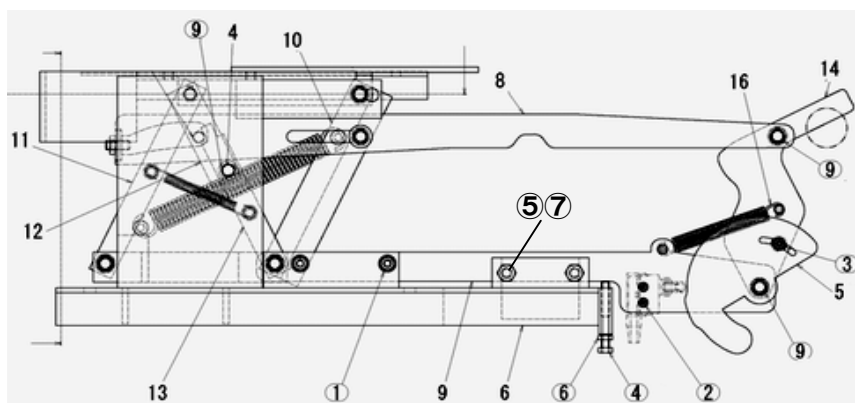
図番7-2-13 DリンクAS
