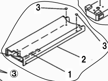
図番13-4-02-4 スライドアームBAS
