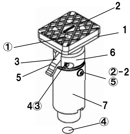
図番37 イージ-アタッチメントHB AS
