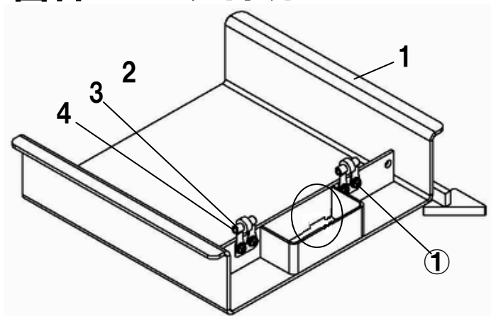
図番15 スライドカバー-RAS
