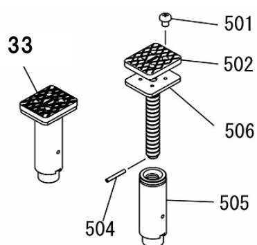
図番33 フレームアタッチメントHB
