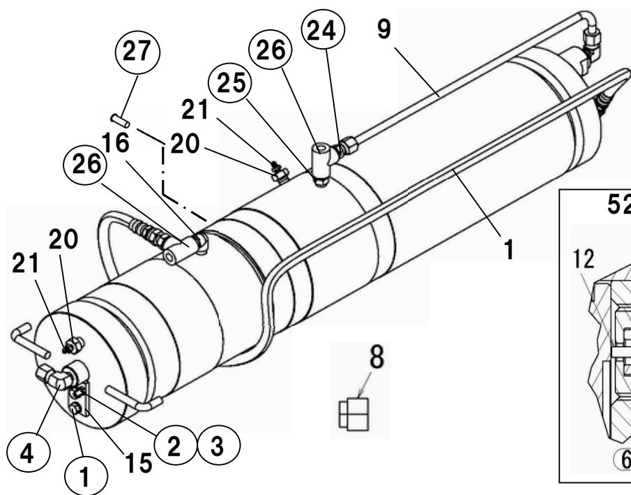
図番52-6 別置式シンクロシリンダAS
