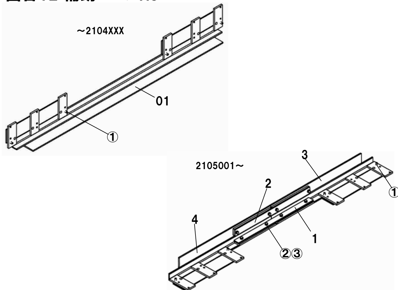
図番12 補助ベースAS
