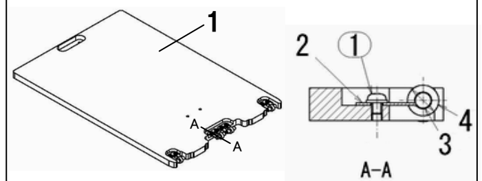
図番5-3 スライドプレートAS
