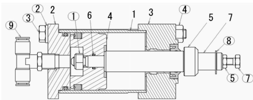
図番7-3-4 爪外しシリンダAS
