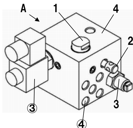
図番8-10 サブプレートAS
