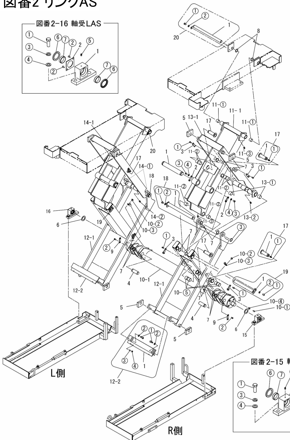
図番2 リンクAS
