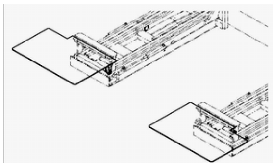
図番4 スライドカバーAS
