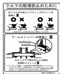
図番 7 11249060 コーションシールH (170mmX120mm) (1枚)
