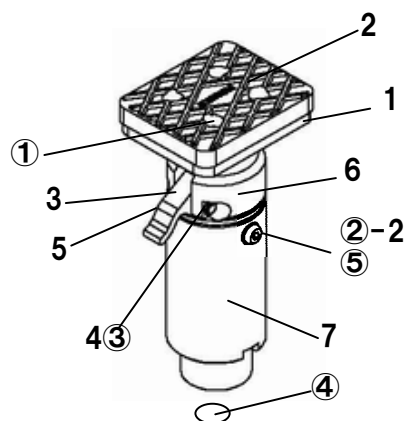
図番27 イージーアタッチメントHB AS
