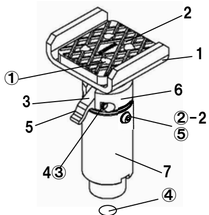
図番26 イージーアタッチメントHA AS
