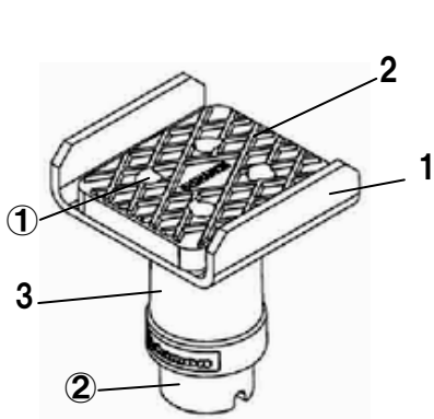
図番40 ライトフレームアタッチメントLA AS
