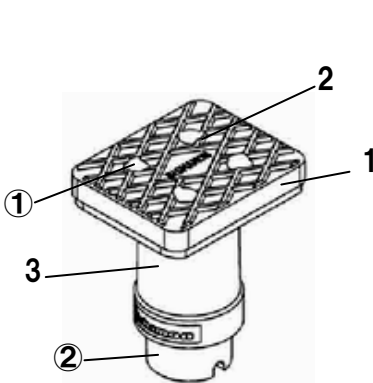
図番41 ライトフレームアタッチメントLB AS
