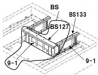
図番 BS132 トラス代替HセットAS
