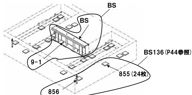
図番 BS129 トラス代替FセットAS
