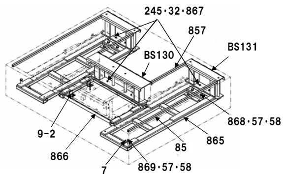
図番 BS135 トラス代替KセットAS
