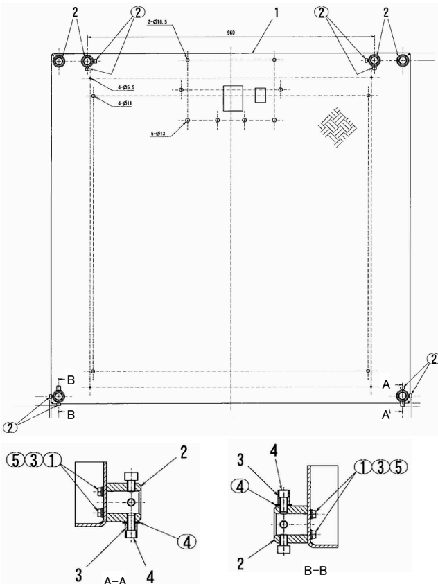
図番8-1 天板AS
