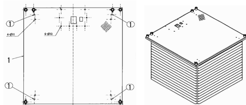
図番8 カバーAS
