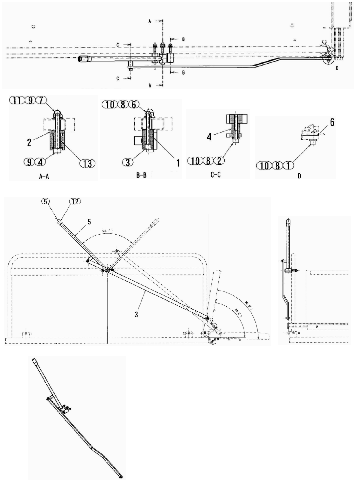
図番12 上階レバー支点AS
