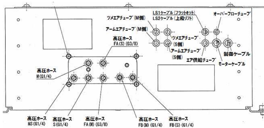
C方向詳細図 (ケーブル接続位置説明図)
