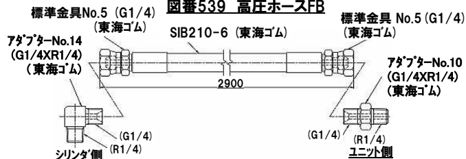
図番539 高圧ホースFB
