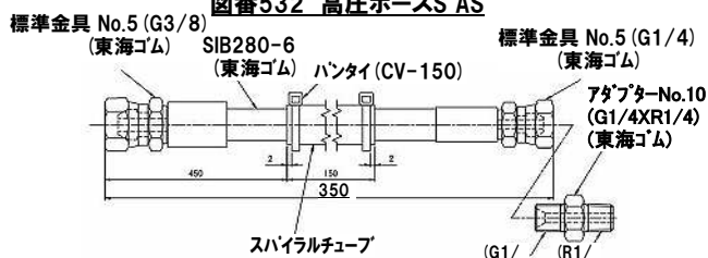
図番532 高圧ホースAS
