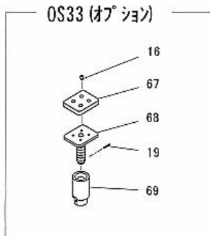
図番74 イージ-アタッチメントLB AS
