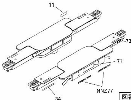
図番73 11516680 コーションシール 90mm×25mm (2枚)
