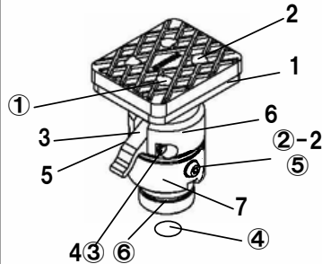
図番74 イージ-アタッチメントLB AS
