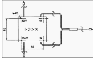
図番585 トランス接続方法
