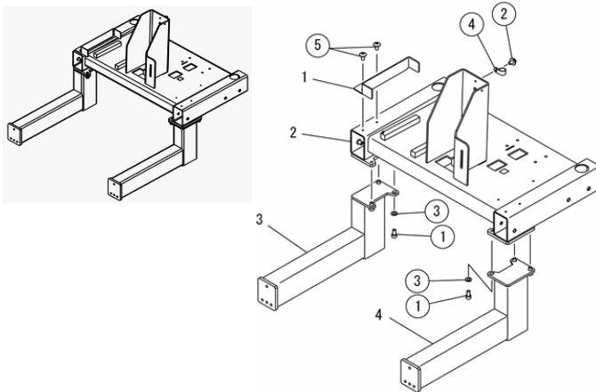
図番3-2 ベースAS
