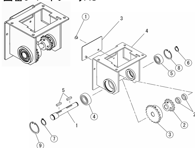
図番3-4 下プーリAS
