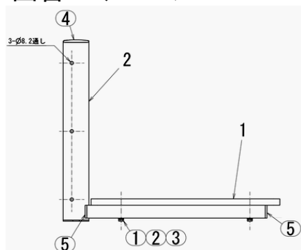
図番6 移動ハンドルAS
