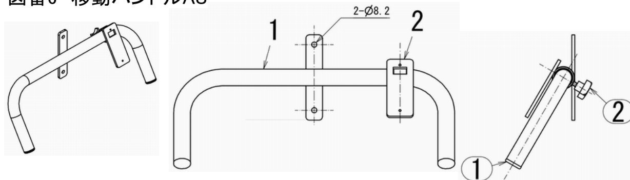
図番6 移動ハンドルAS
