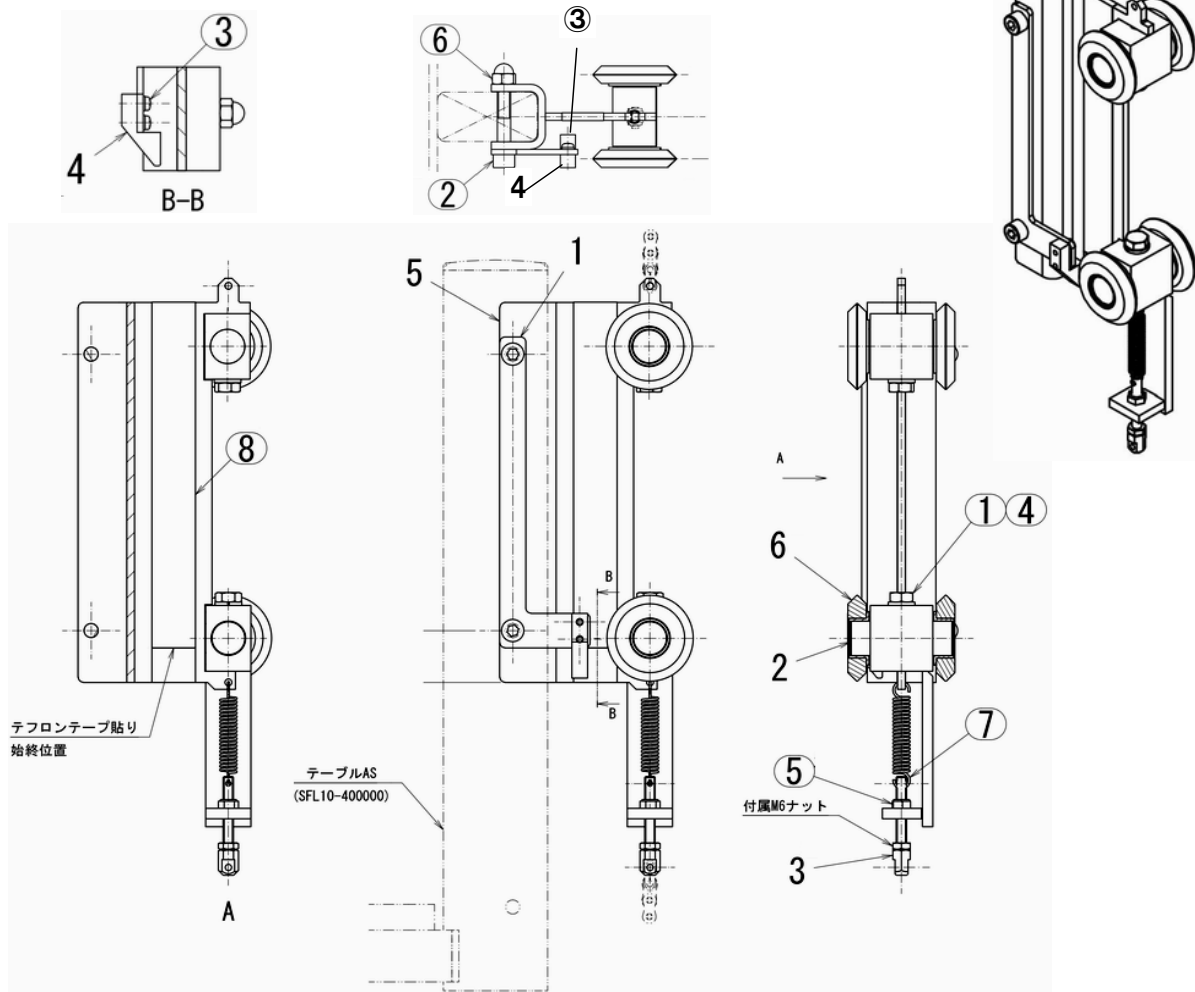
図番5 テーブルAS
