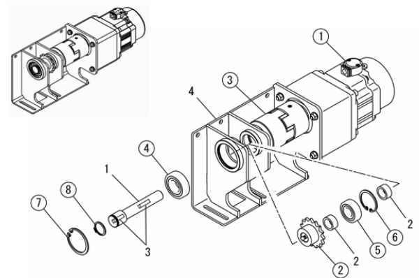
図番3-3 モータAS
