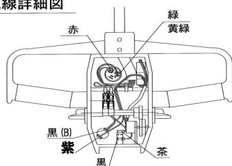
ケーブル詳細図
