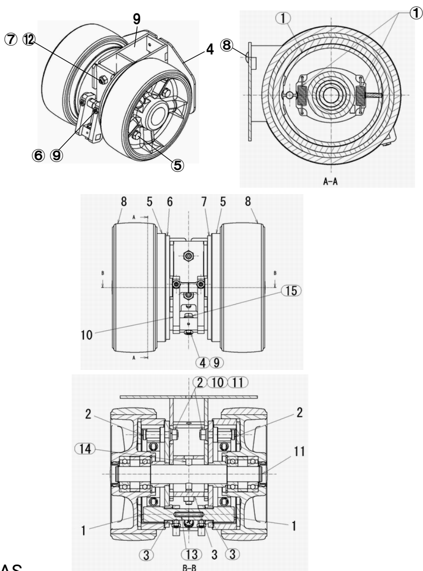
図番5-4 ブレーキ本体AS
