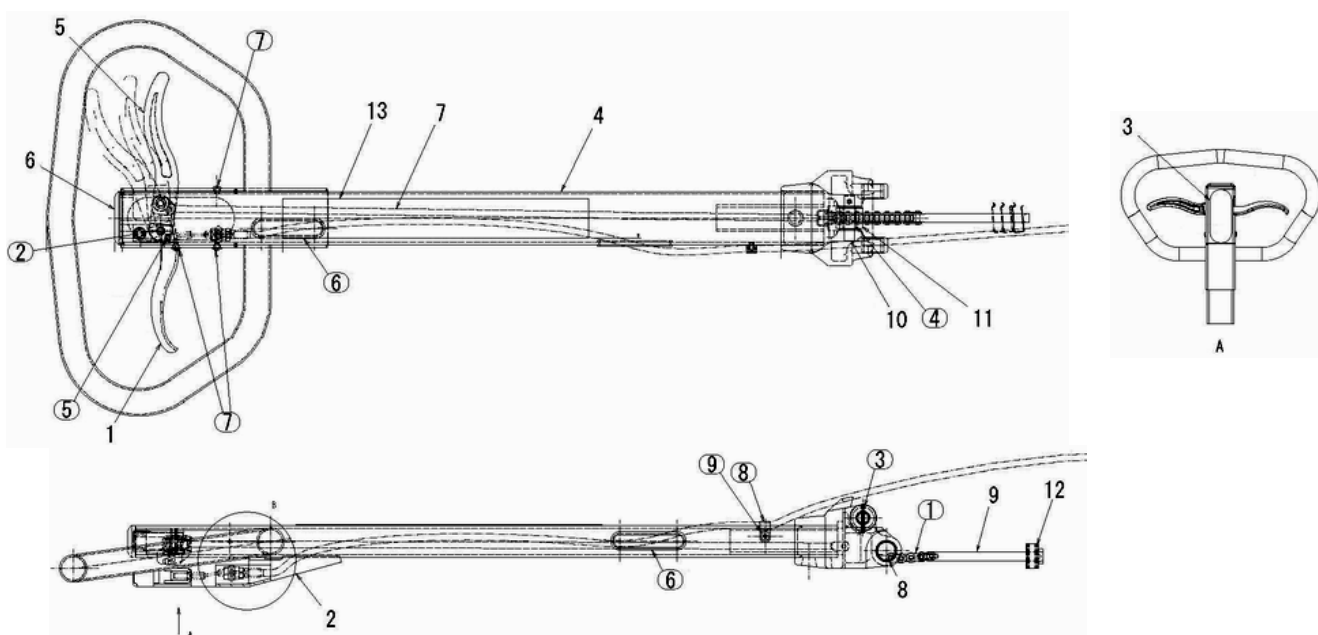
図番5-5 ブレーキハンドルAS
