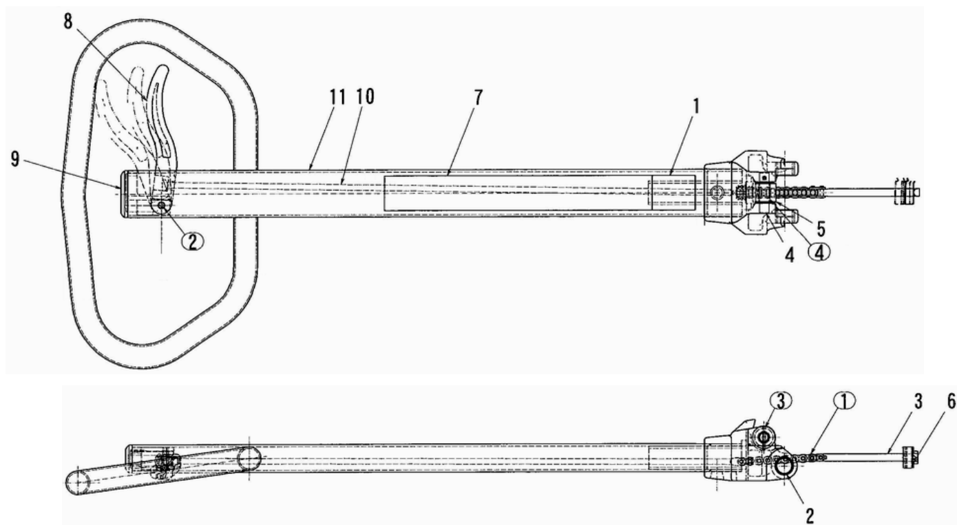
図番4-2 鉄ハンドルAS
