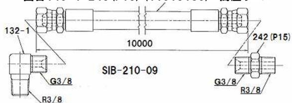
図番140-2・450 (P19) (11019181) 高圧ホース
